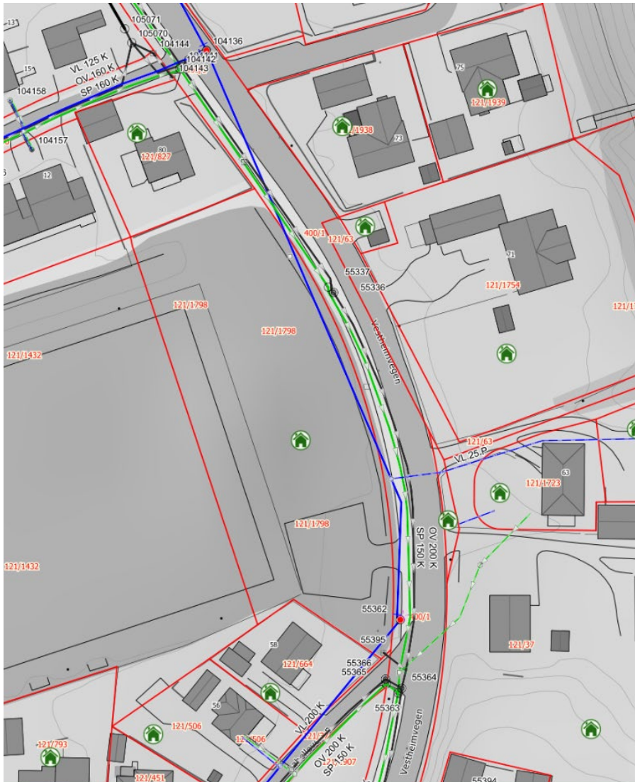
Figur 29, VA-ledninger, kilde: Porsgrunn kommune, blå linje er vannledning VL200.
