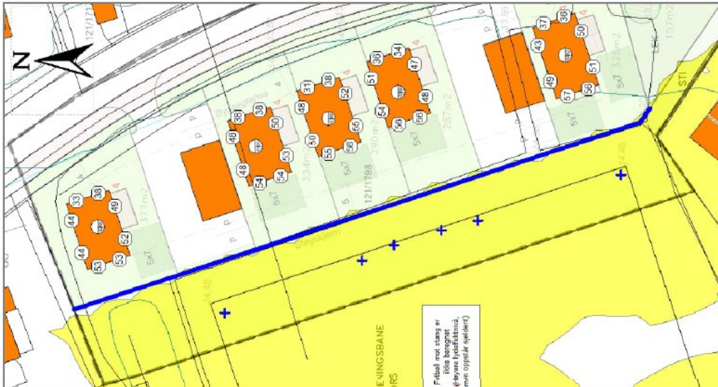
Figur 35, Akustikk-konsult AS, Støysonekart: Støyskjerm mellom nye boliger og idrettsanlegget. Maksimalt støynivå LAFmax fra fotballbanen. Beregningshøyde 1,5 meter over bakken for uteoppholdsareal. Fasadenivåer for 1. etasje er markert på bygningene. Blå kryss representerer de mest utsatte punktene på banen, og viser hvor støykildene er plassert i modellen. Gul støyzone markerer støynivå over 60 dB.
