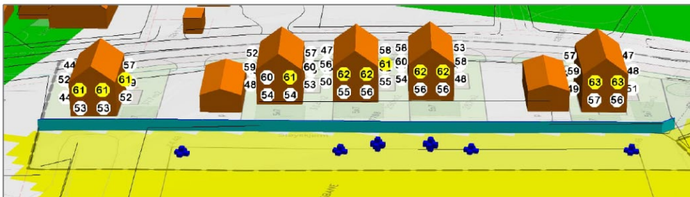
Figur 36, Akustikk-konsult AS, Støysonekart: Støyskjerm mellom nye boliger og idrettsanlegget. Lydnivå LAFmax på fasader fra fotballbanen, sett fra vest.
