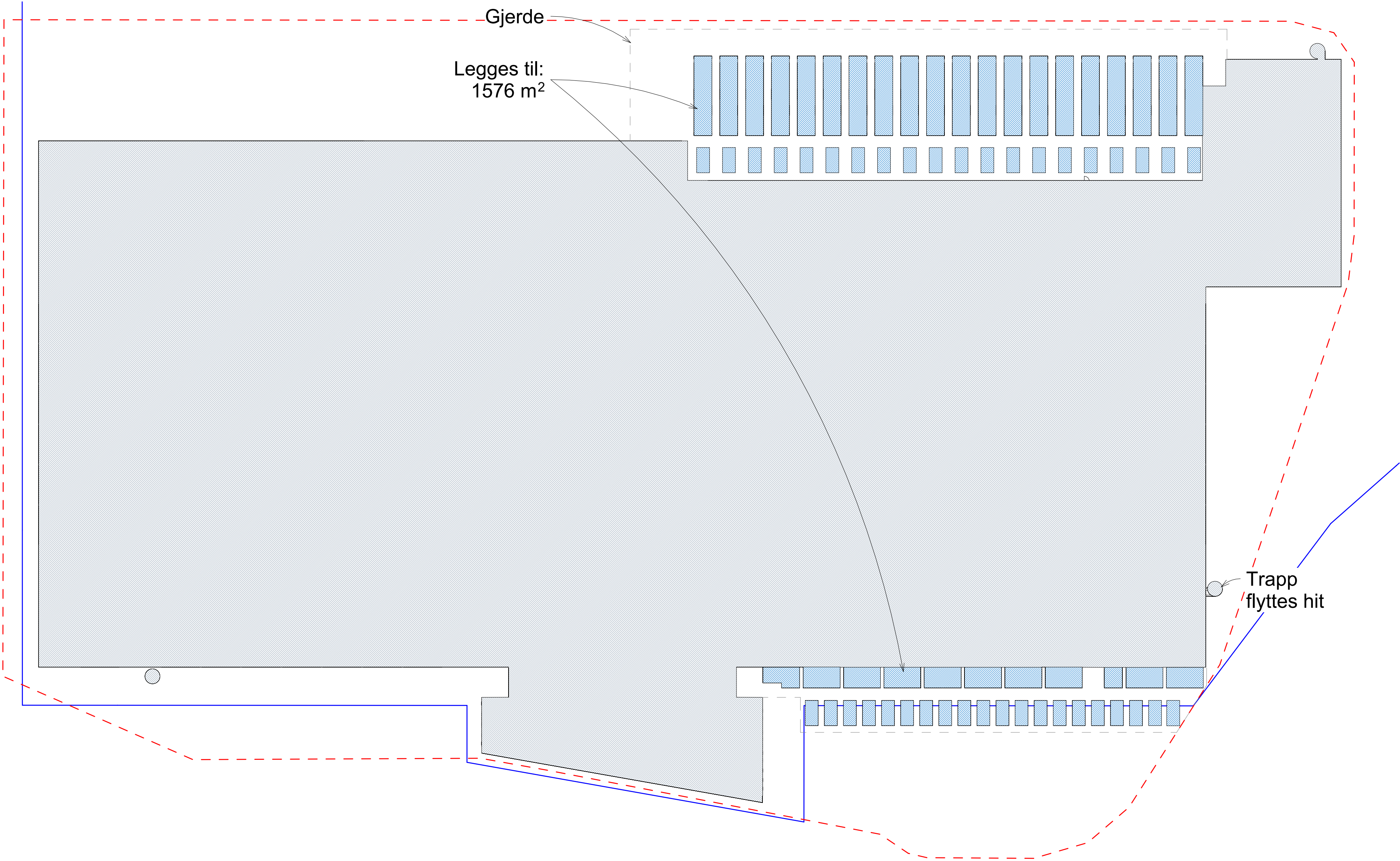
2 BYA ny 1 : 500
