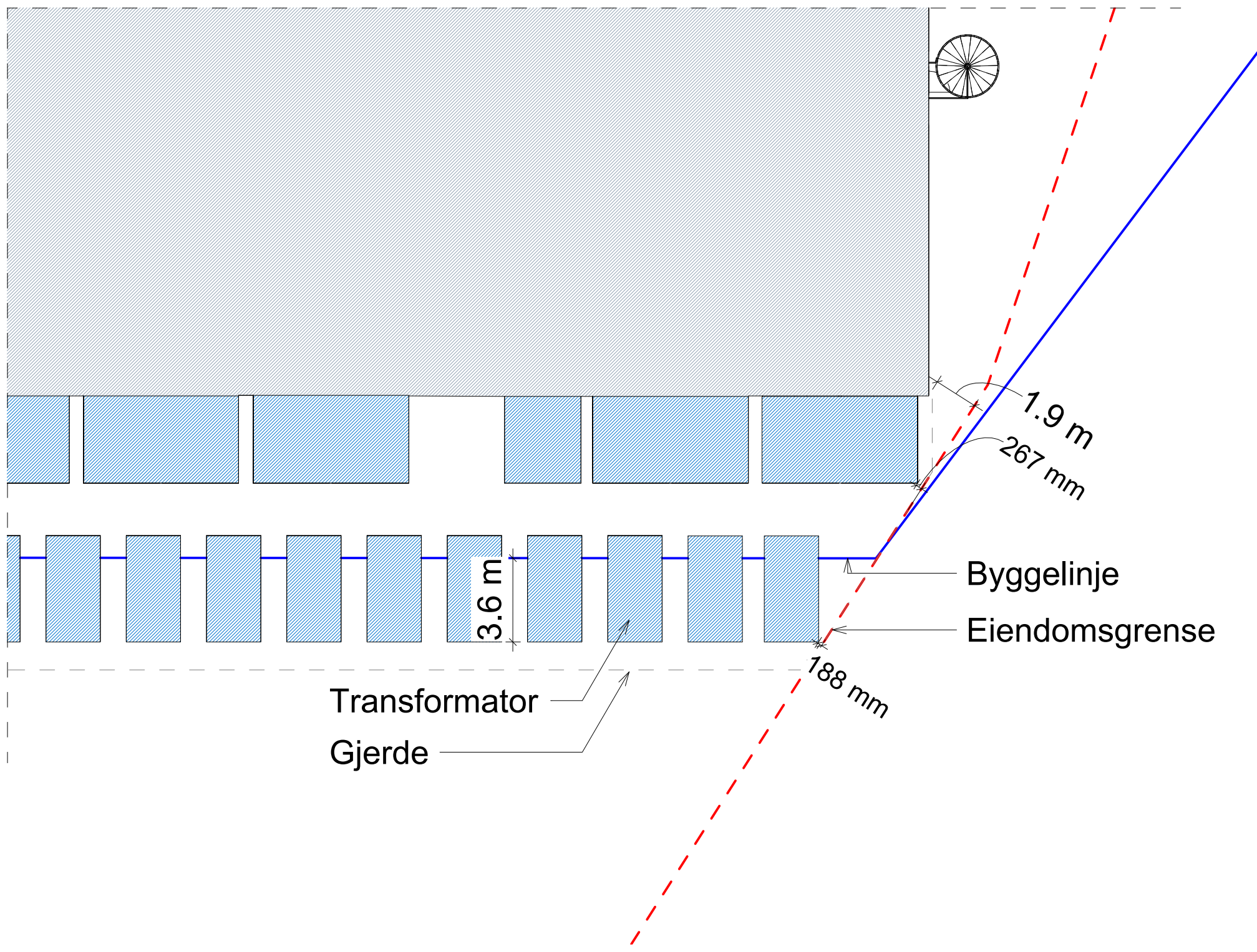
3 Avstander 1 : 200
