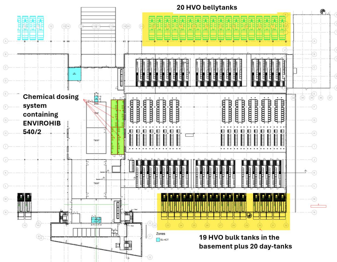
Figur 2: De identifiserte stedene for lagring og bruk av farlige stoffer på tegningen som viser den østlige delen av området, i bygg 624. Stedet for kjemisk dosering er vist i lysegrønt, HVO-dieseloljetankene med gul markering.
