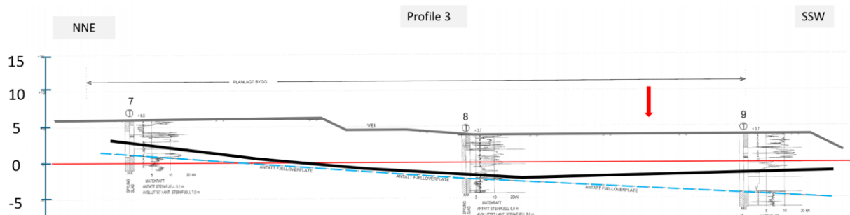
Figur 34: Det gjengitte tverrsnittet 3 (traseen er angitt i Figur 31) fra 2007 fra den geotekniske rapporten [11], med loggede totalsonderinger i borehull, og med AFRYs tolkning av formasjonsgrensene. Den stiplede lyseblå linjen er toppen av berggrunnen, den svarte linjen er toppen av marin siltig leire, og den grå linjen representerer terrengoverflaten. Det øverste laget mellom den grå og den svarte linjen er forurenset fyllmasse. Den tidligere strandlinjens posisjon i tverrsnittet er vist med en rød pil. Den vertikale skalaen er meter under og over havnivå. Havnivået er angitt med en rød linje.
