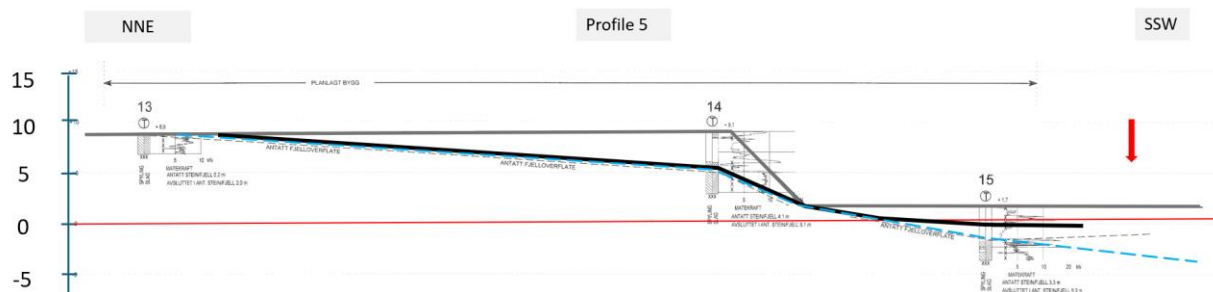
Figur 36: Det gjengitte tverrsnittet 5 (traseen er angitt i Figur 31) fra 2007 fra den geotekniske rapporten [11], med loggede totalsonderinger i borehull, og med AFRYs tolkning av formasjonsgrensene. Den stiplede lyseblå linjen er toppen av berggrunnen, den svarte linjen er toppen av marin siltig leire, og den grå linjen representerer terrengoverflaten. Det øverste laget mellom den grå og den svarte linjen er forurenset fyllmasse. Den tidligere strandlinjens posisjon i tverrsnittet er vist med en rød pil. Den vertikale skalaen er meter under og over havnivå. Havnivået er angitt med en rød linje.
