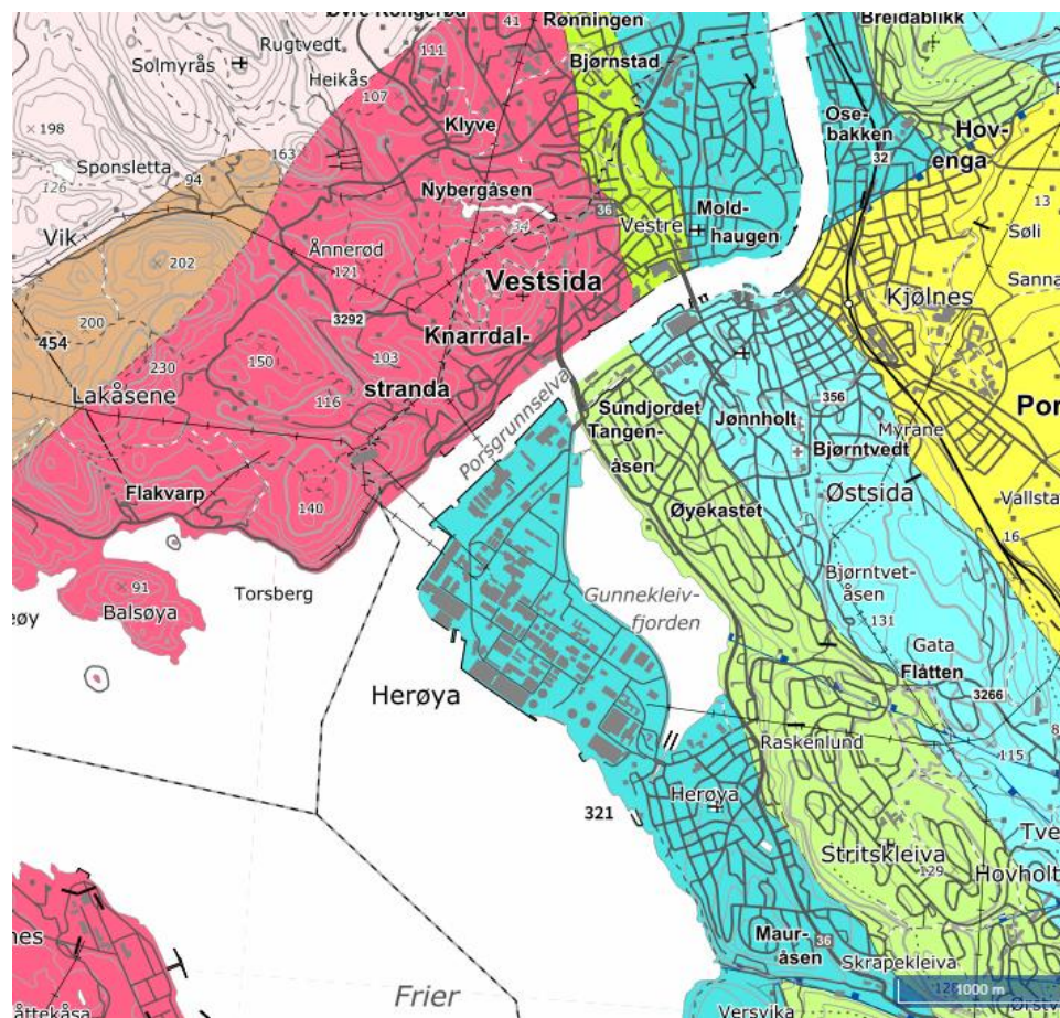
Figur 3: Berggrunngéologisk kart av området rundt Herøya. Herøya er en del av, og ligger på kanten av Oslo-grabenen, og består av paleozoiske karbonatbergarter. Kilde: www.ngu.no
