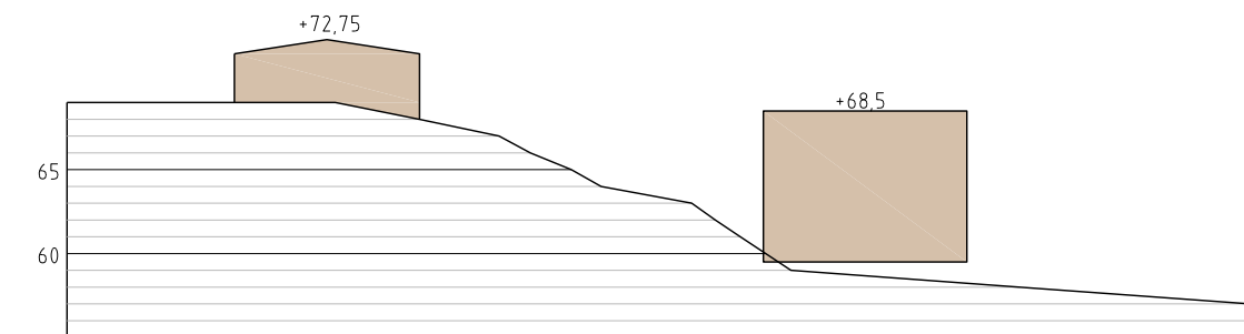
Snitt D
