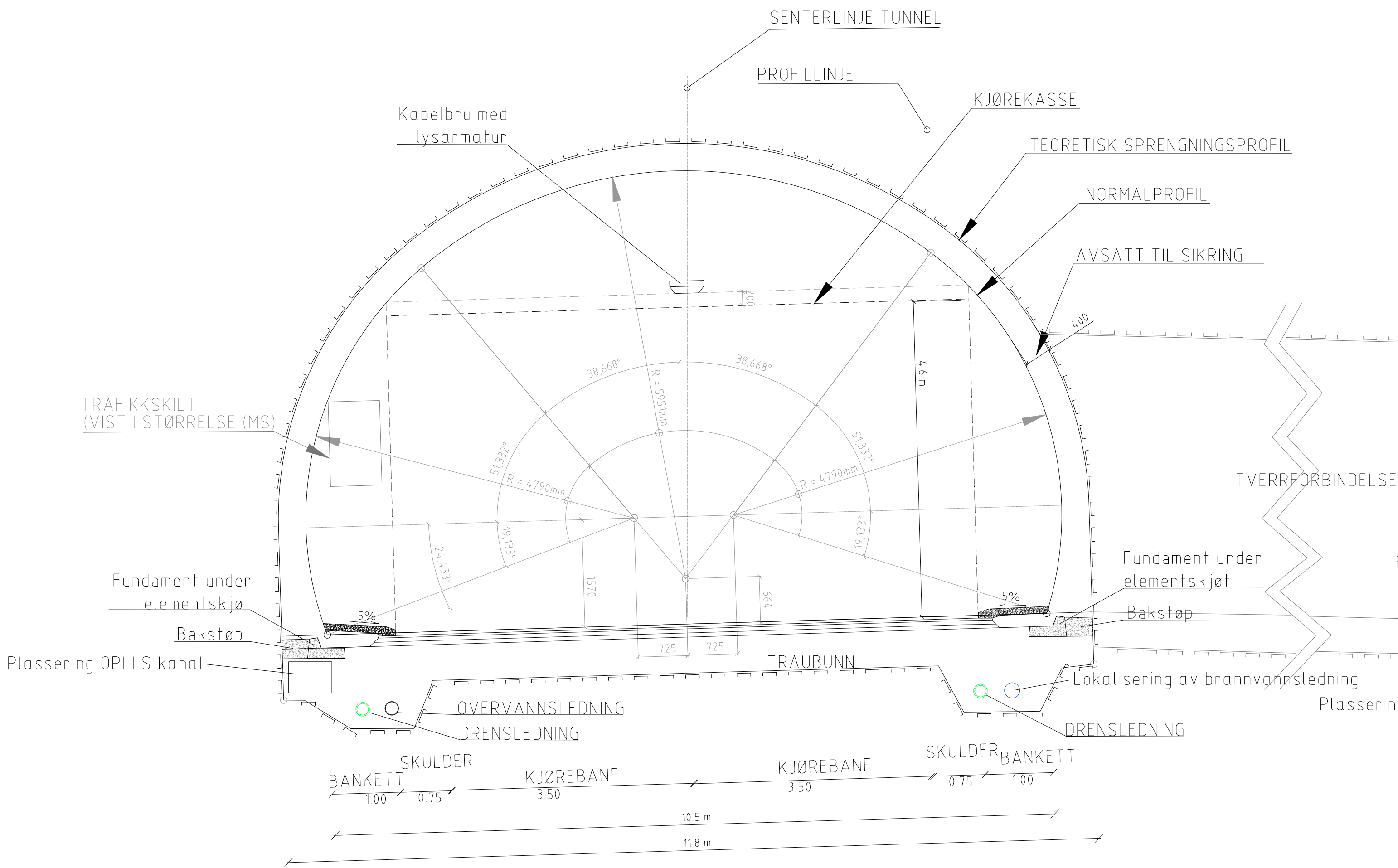
Normalprofil E18 (mot kjøreretningen) - T10.5 Profil med 2 grøfter
