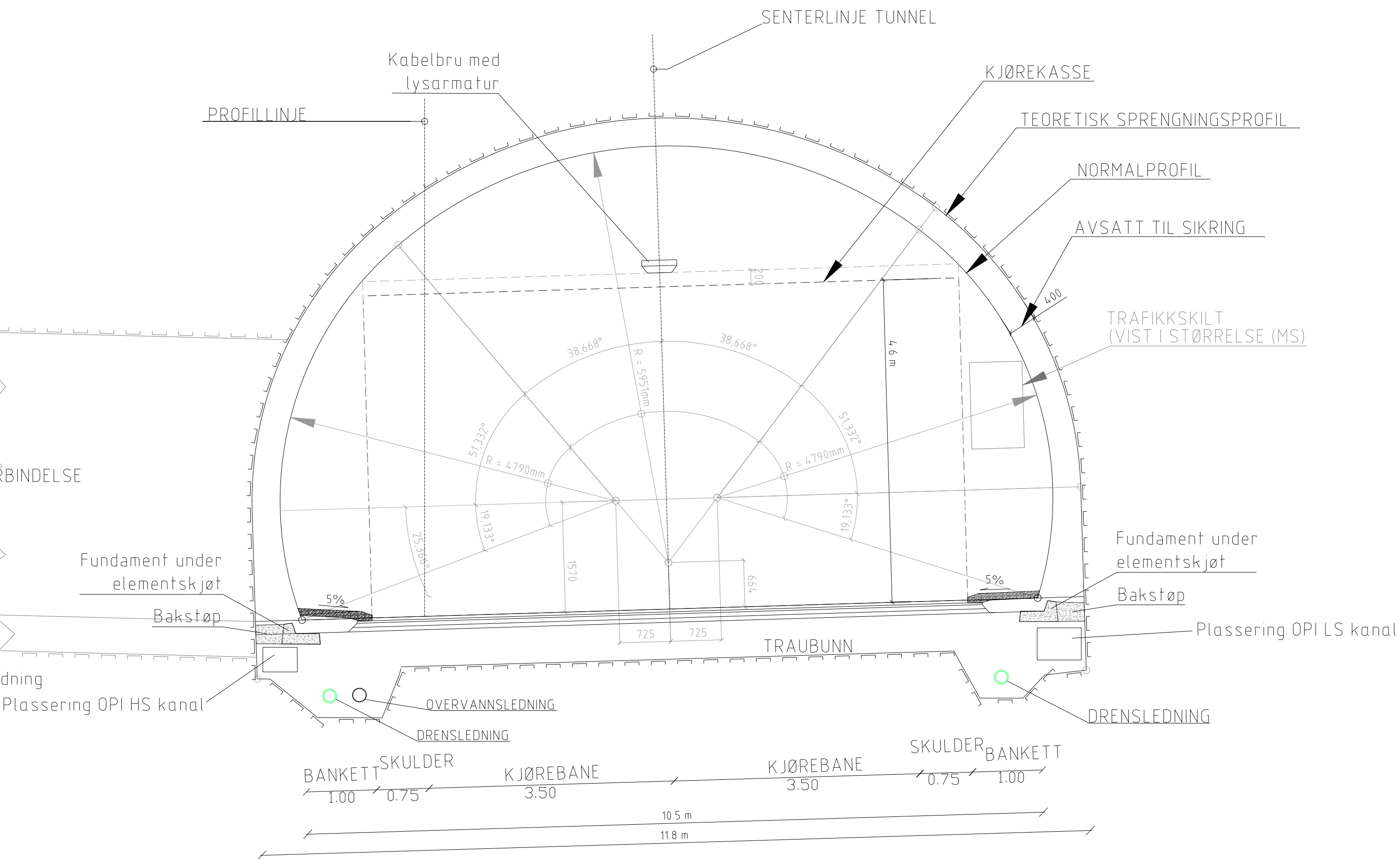
Normalprofil E18 (med kjøreretning) - T10.5 Profil med 2 grøfter
