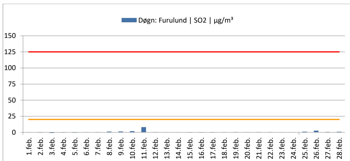
Figur 7: SO 2 ved Furulund målestasjon
