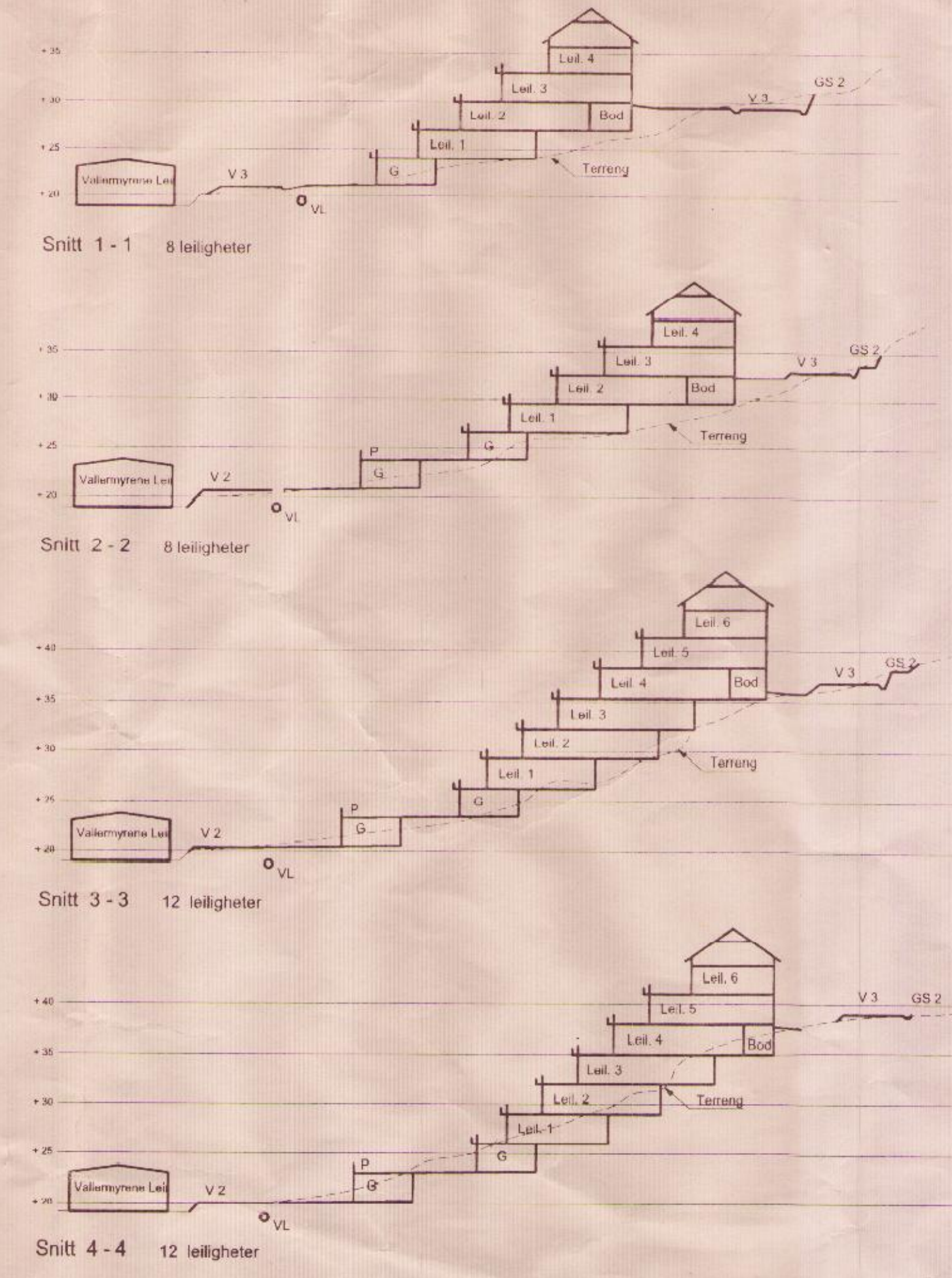
Illustrasjonssnitt for terrasseboliger område B 9 Målestokk 1 : 500
