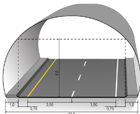
Figur 3-2 Tunnelprofil T10,5 (mål i meter)
