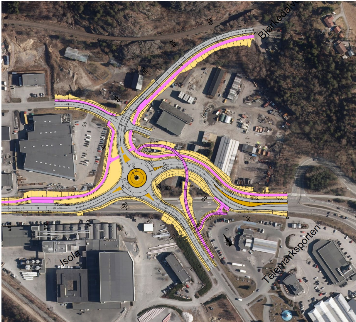
Figur 2 Forslag til kryssombygging
