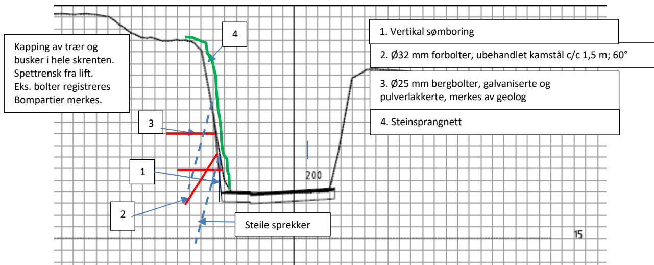
Figur 11c. Tverrprofil 200 med sømboret vertikal skjæring med ansett midt i bergveggen. På grunn av slepper med fall inn i skjæringen, vil det være lokale overheng som gjør vertikal sømboring vanskelig. Det kan bli nødvendig å foreta mindre sprengingssalver i bunn av ny skjæring supplert med horisontal boring langs prosjektet skjæring.
