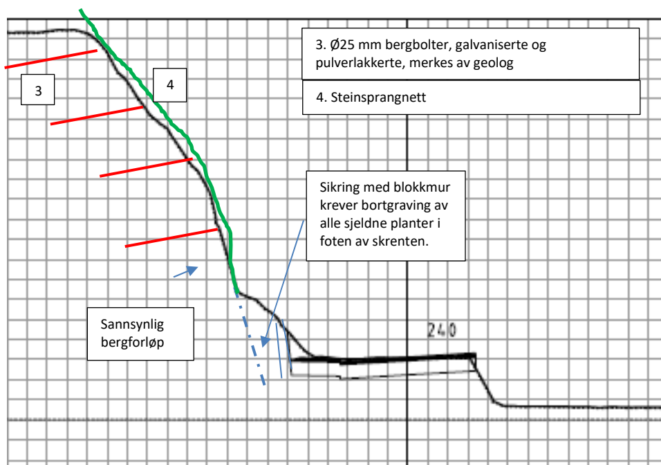
Figur 11d. Tverrprofil 240. Vegetasjonsrens og spettrensk skal utføres før bolting og montering av nett. Sikringsentreprenør skal påse at renskemasser ikke kan føre til skade på bolig i Strømtangveien 18. Biolog skal godkjenne kapping av trær i topp av skrent og bortgraving av sjeldne planter i foten av skrenten før utførelse.
