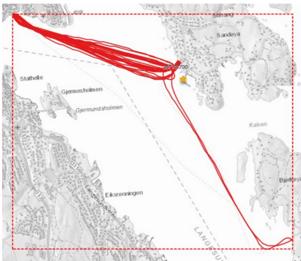
Figur 1: seilingsmønster Breviksferga i dag vist med røde streker. Ny fergekai vises med gul stjerne. (kilde: Brevik fergeselskap)
