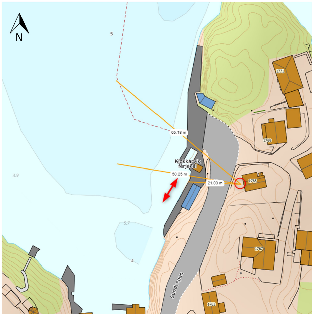
Figur 1: Fergekaien på Klokkarvik. Rød dobbeltpil markerer fergens posisjon ved kai og rød sirkel målepunkt for lyd. Blått rektangulært bygg på kaien er trafo.
